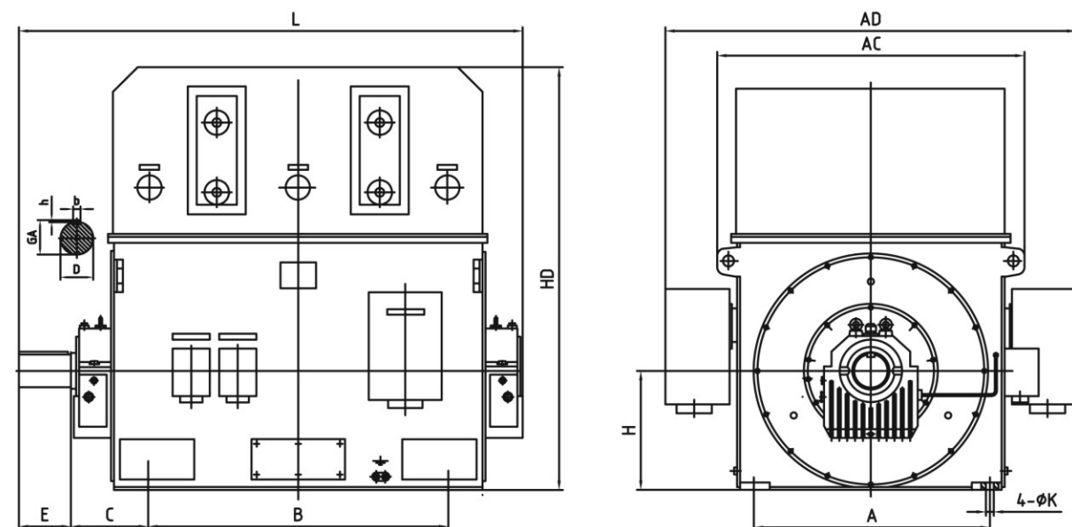
YKS系列大型高压三相异步电动机外形尺寸图
