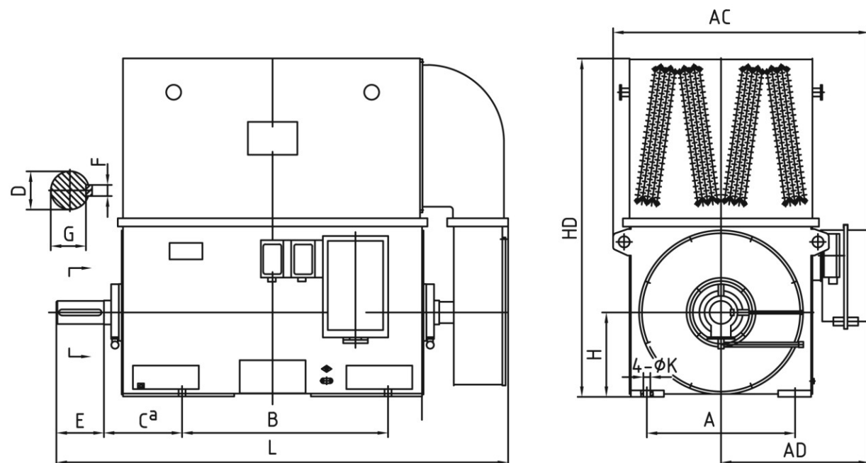
YKK系列 (10kV) 中型高压三相异步电动机外形尺寸图
