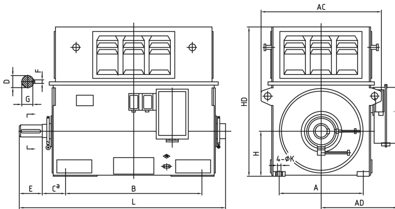
Y系列 (10kV) 中型高压三相异步电动机外形尺寸图
