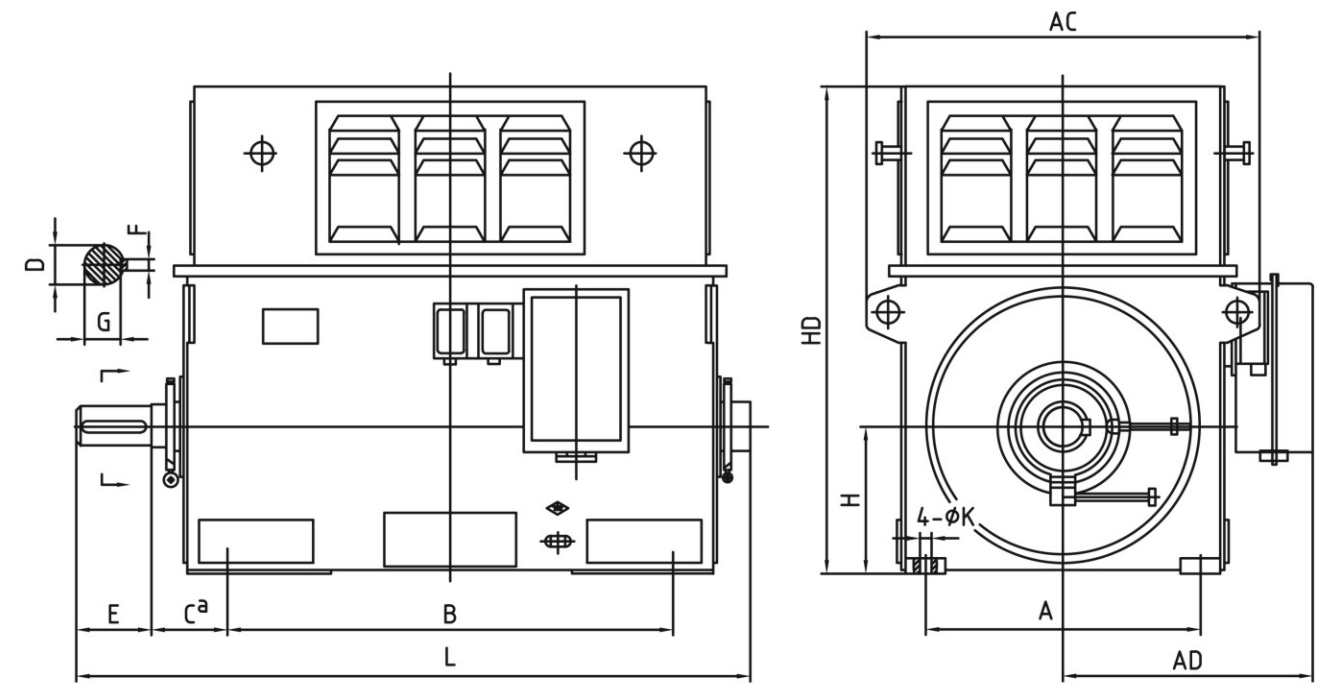
Y系列 (6kV) 中型高压三相异步电动机外形尺寸图
