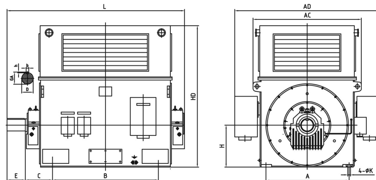
Y系列大型高压三相异步电动机外形尺寸图
