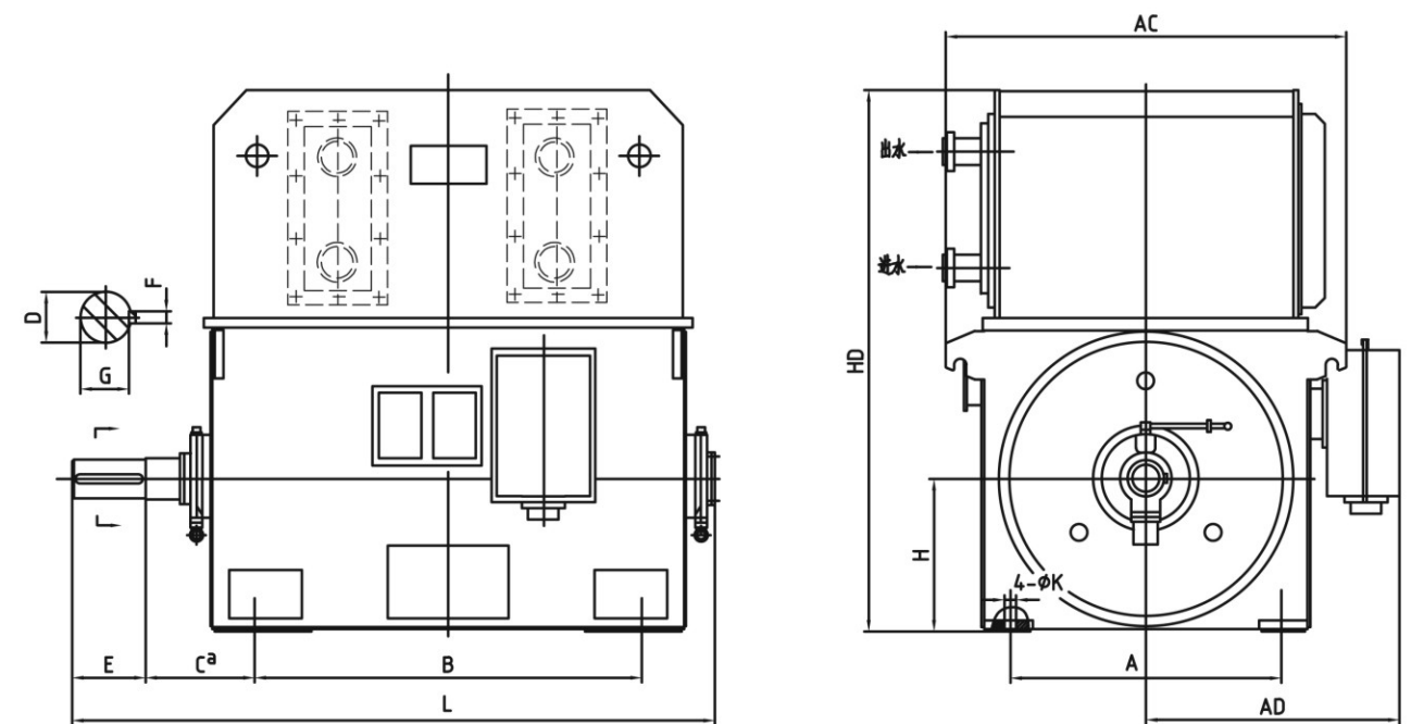
YKS系列 (6kV) 中型高压三相异步电动机外形尺寸图
