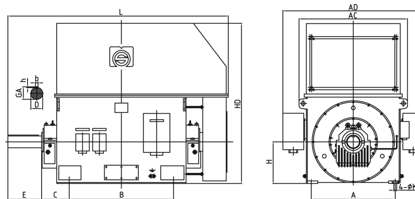
YKK系列大型高压三相异步电动机外形尺寸图
